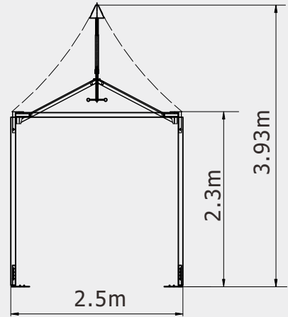
Type M-PAG2.5/230
