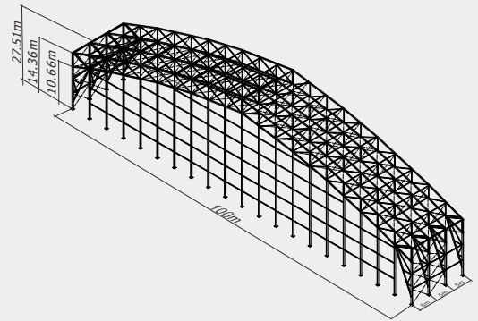
Type : ATS100/1000
